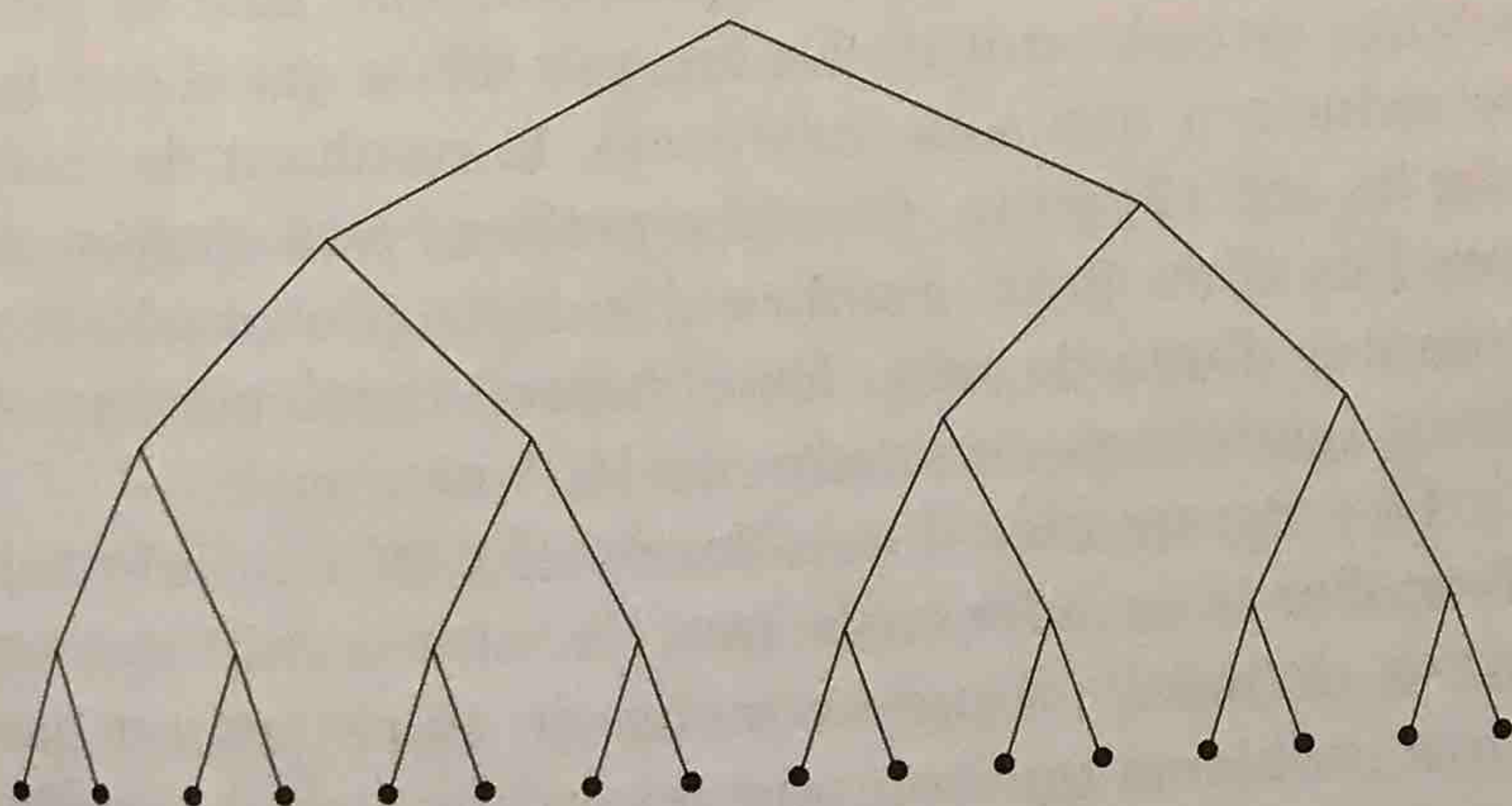
Figura 4: Els estats d'equilibri d'un vidre de spins s'organitzen jeràrquicament ocupant els extrems inferiors d'una estructura d'arbre. L'exemple mostrat correspon a un arbre binari.
