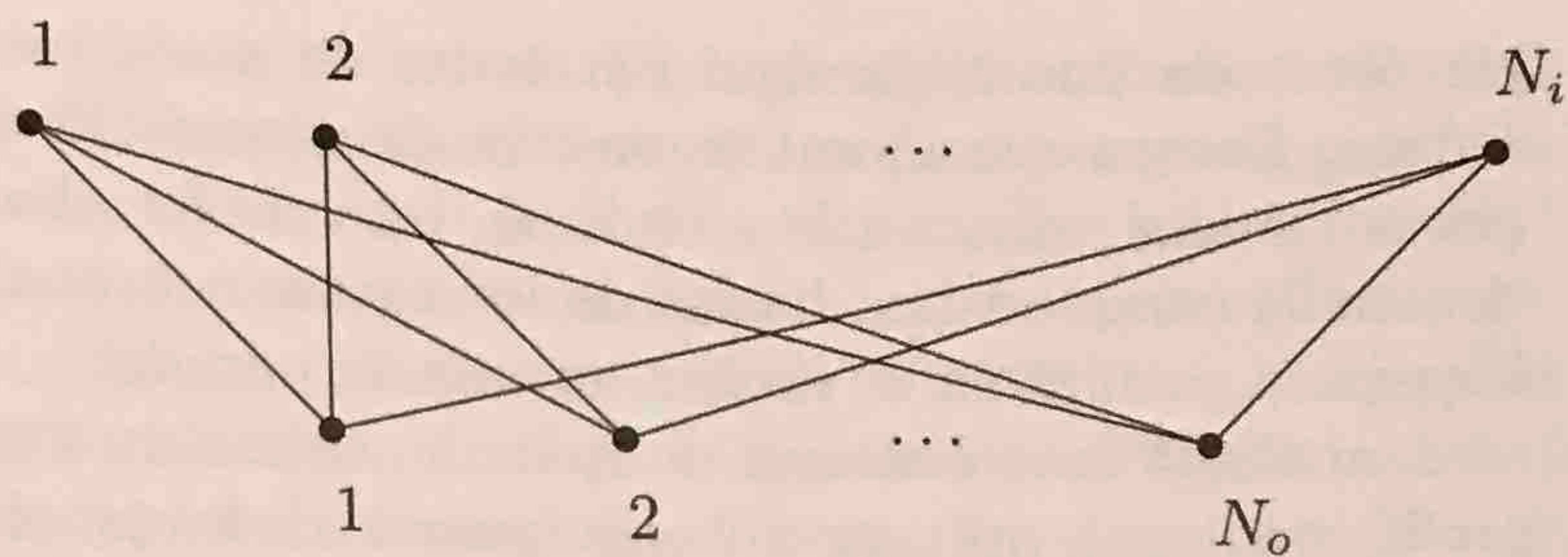
Figura 5: Xarxa feed-forward per a un perceptró de dues capes: entrada de N_i unitats, i sortida de N_o . Les connexions no són dobles, sinó que només tenen lloc en sentit d'entrada a sortida
