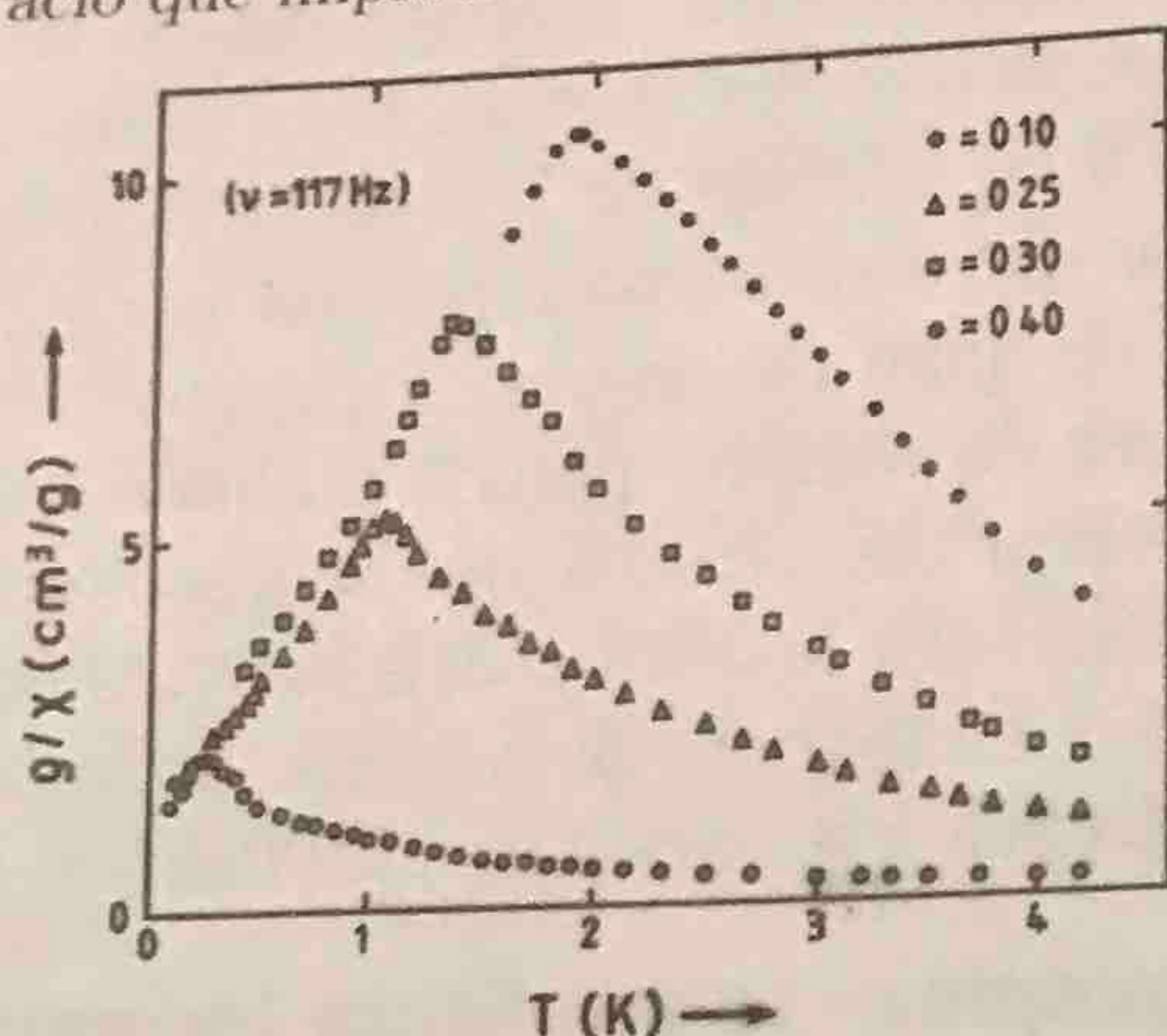
Figura 2: Pic de la susceptibilitat en un vidre de spins metàl·lic. Encara que no hi hagi divergència això és un indicatiu de l'existència d'una transició de fase
