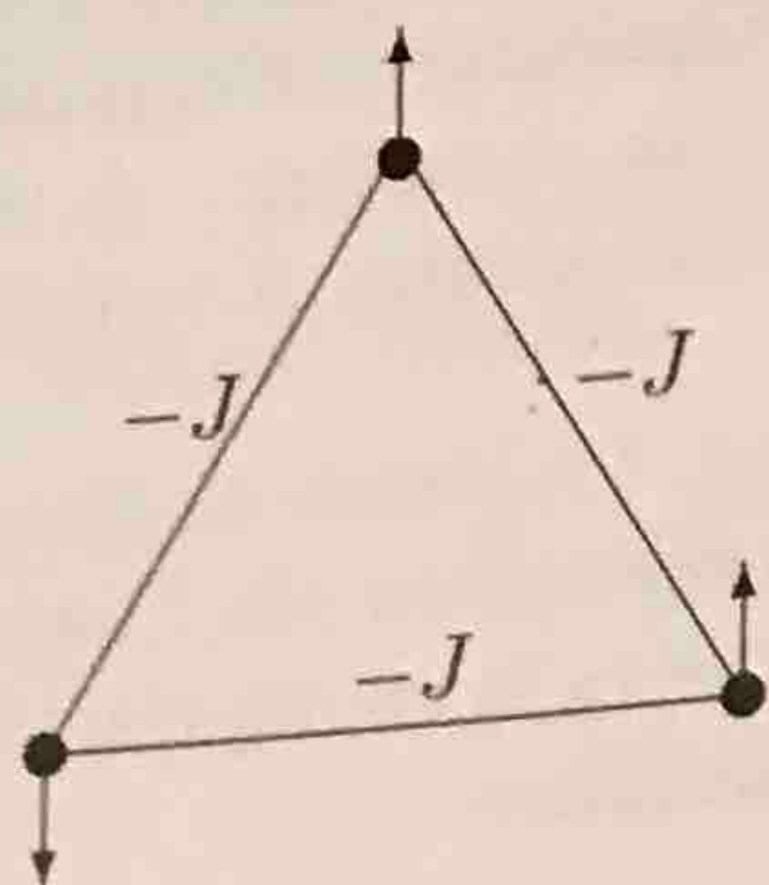
Figura 1: Tres spins frustrats. La unió a la part superior dreta està "insatisfeta". En un sistema macroscòpic hi ha una frustració que implica un nombre molt elevat de spins
